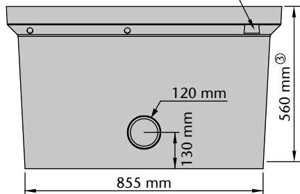
Optional riser
